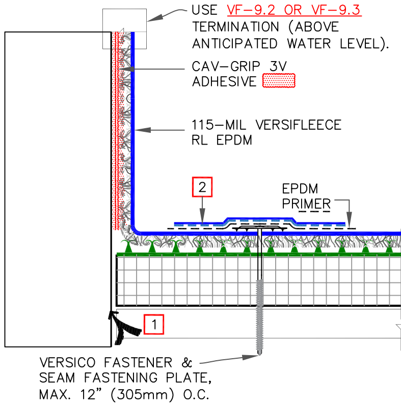
OPTION A (CAV-GRIP 3V & RL MEMBRANE)
